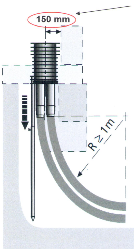
Reiheninstallation 4-fach
