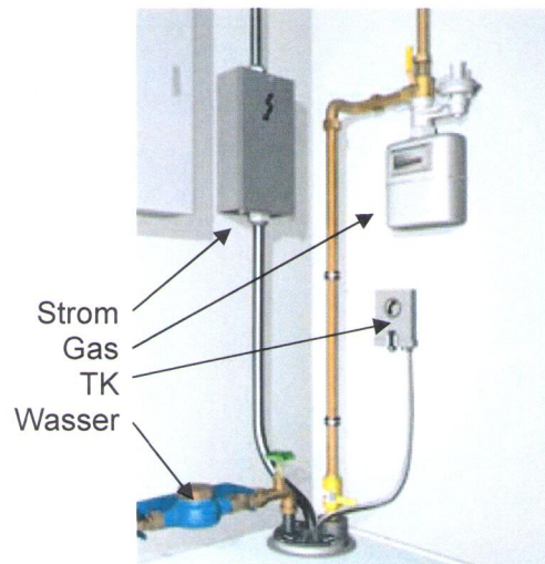
Beispieldarstellung für die Anordnung der Übergabestellen
