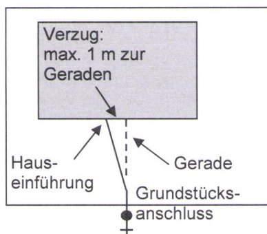
Leitungsverzug max. 1m
